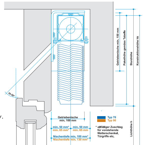
Vertikalschnitt mit Hohlsturz
