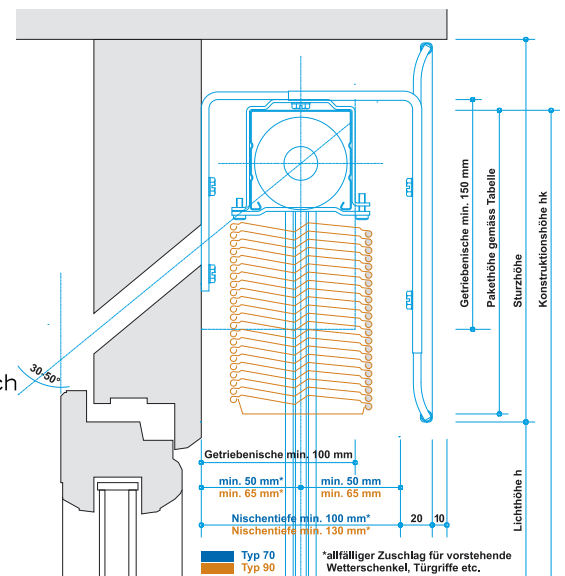
Vertikalschnitt mit Blende
