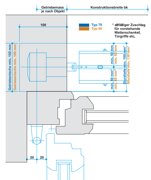
Horizontalschnitt
